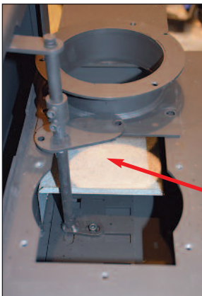
Ansicht des im Bereich des Zuluftanschlusses an der Brennkammer werkseitig eingebauten Schmutzfangbleches. Dient zum Schutz des Zuluftreglers gegen evtl. herabfallende Kehrreste aus dem Zulufschacht.
